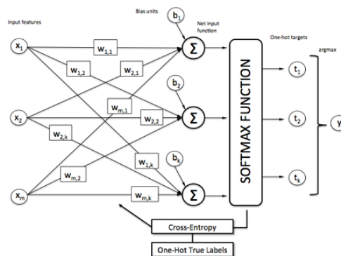
Fig. 5: Softmax classifier.
