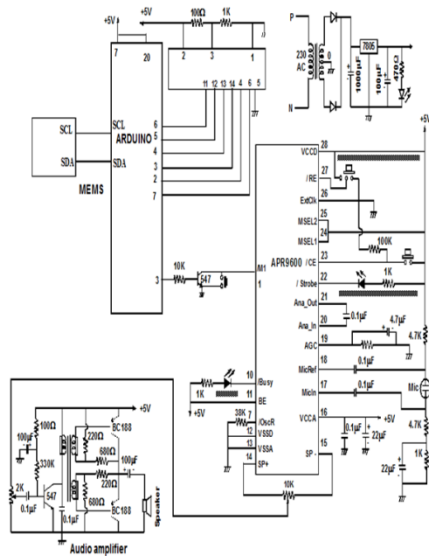
Fig. 3.: Circuit Diagram
