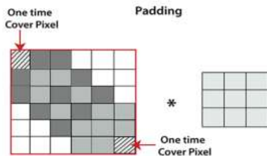
Fig 6. Padding structure
