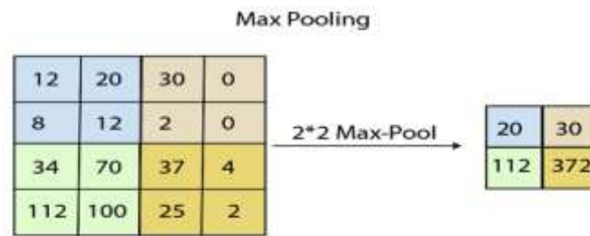
Fig 7.Pooling layer
